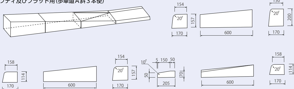
セーフティ及びフラット用(歩行道A斜3本使)
