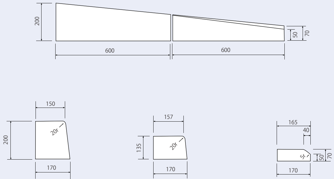
都型A 1 (右・左)
