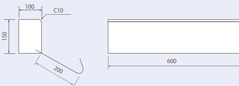
100×150×600 (鉄筋出し)
