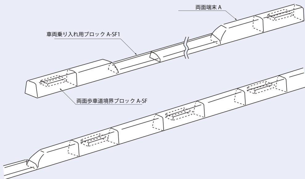
施工図
