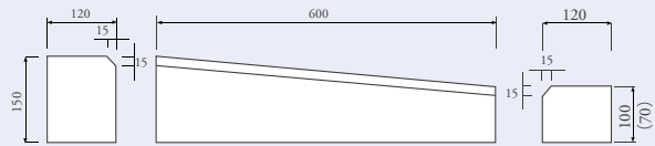
地先境界ブロックB平10cm(7cm)
