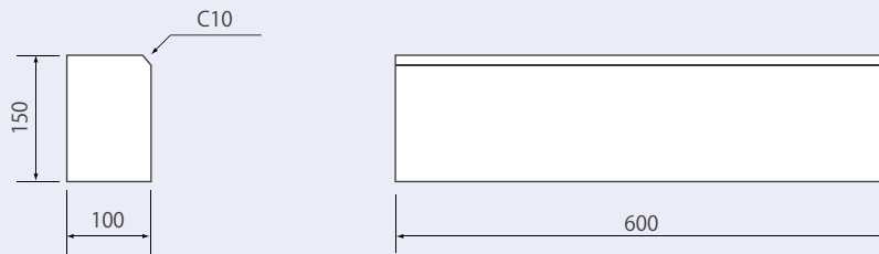
100×150×600
