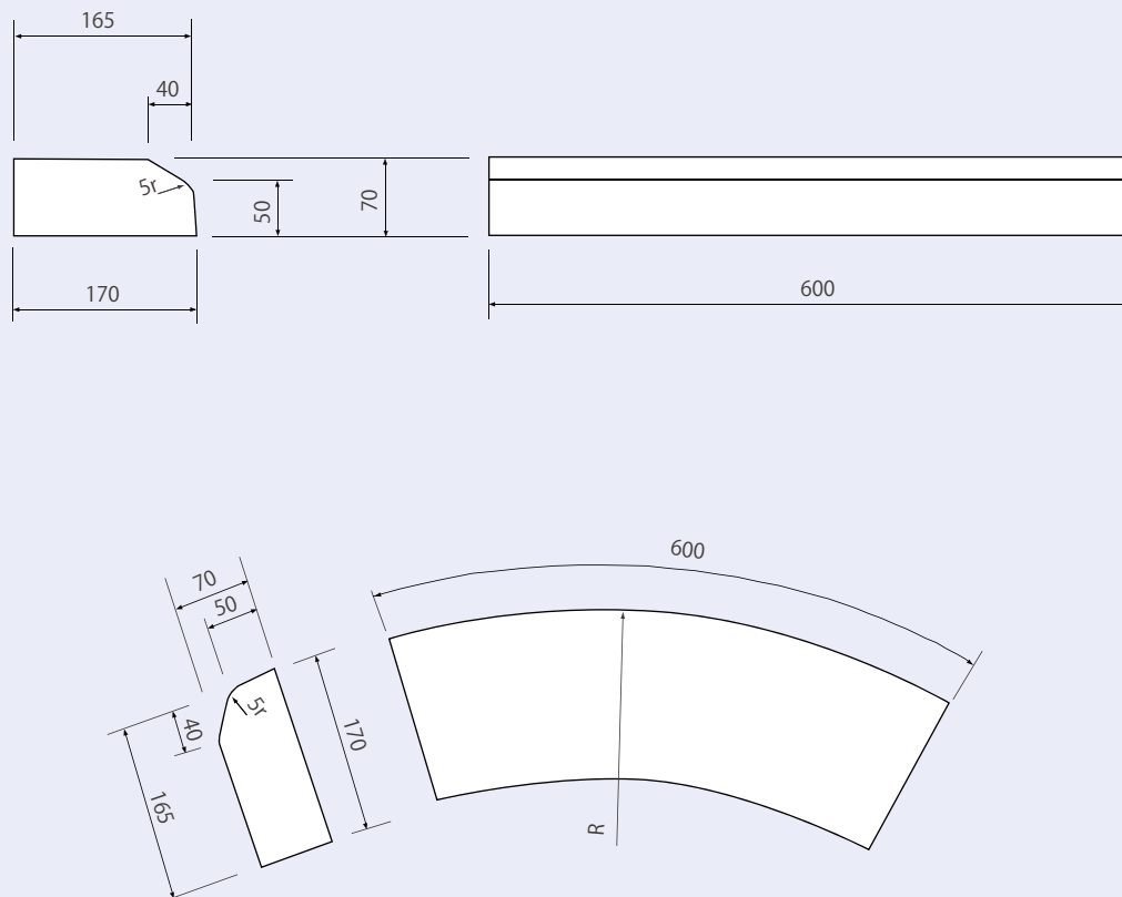
中央区型C 1
