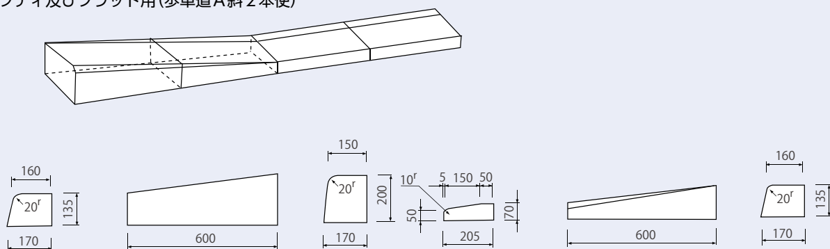
セーフティ及びフラット用(歩行道A斜2本使)
