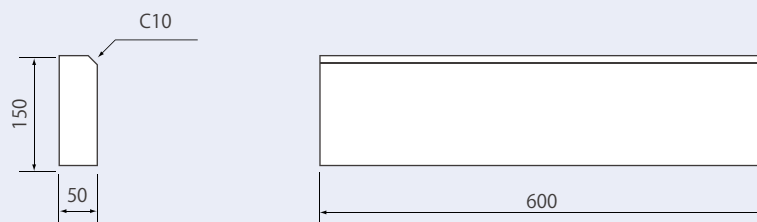
50×150×600 (半コーピンタイプ)
