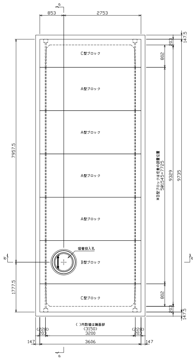
基礎図(※1) (鉄筋コンクリート)
