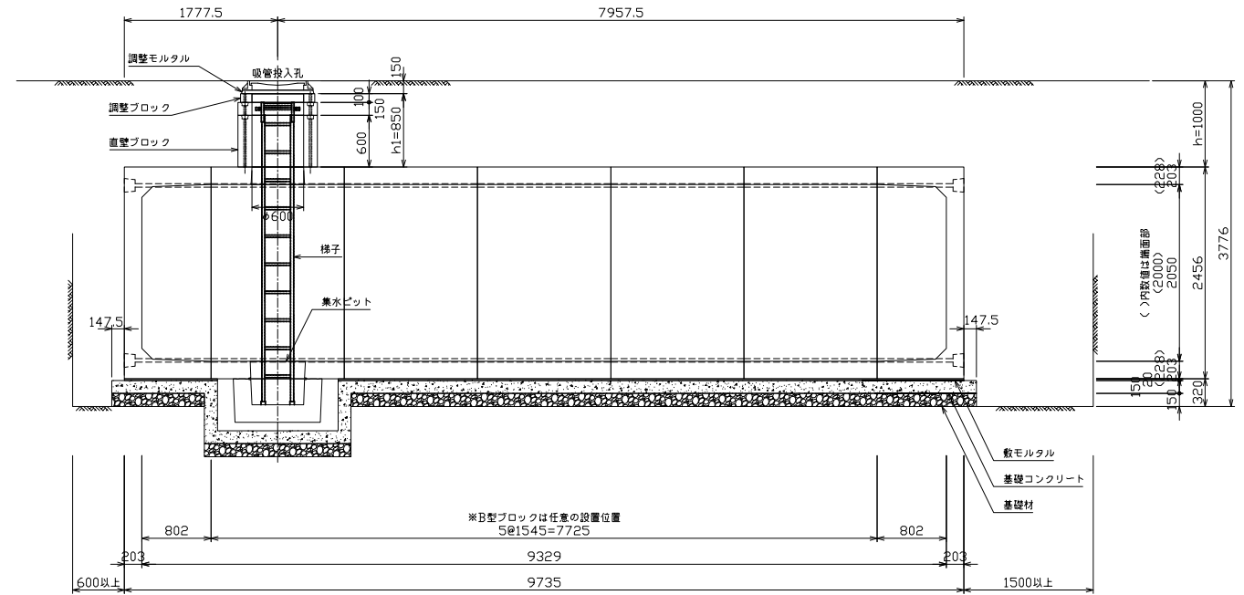
a-a断面図
