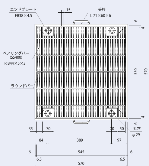
グレーチング細目タイプ
