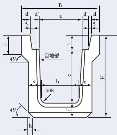
目地部詳細図
