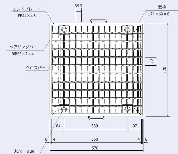
グレーチング標準タイプ
