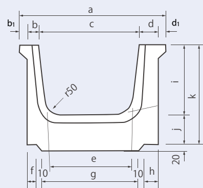
上部側塊
