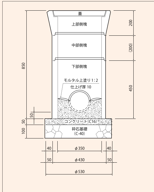
組立図
