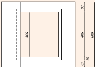
街渠柵 155用縁塊
