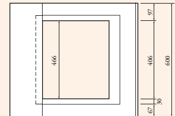
(歩道用)
