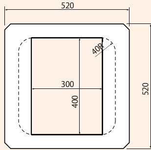
上部側塊
