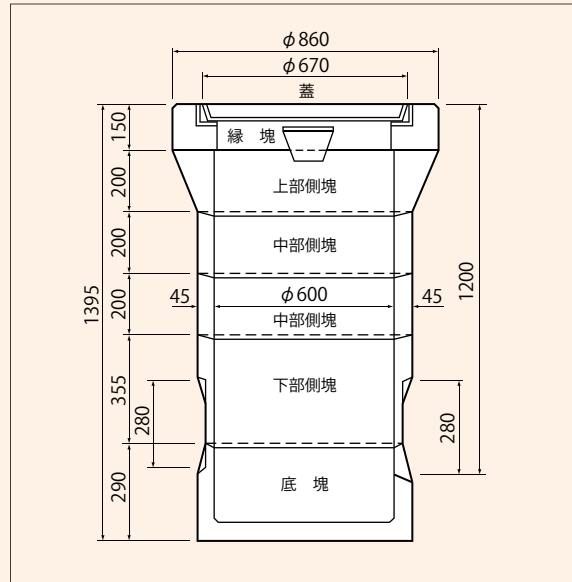
組立図 雨水
