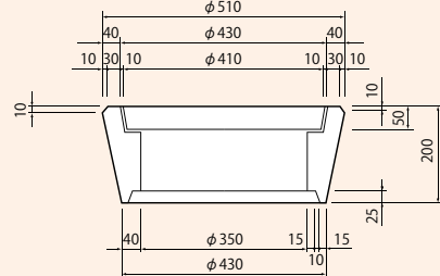
蓋 (T-14)
