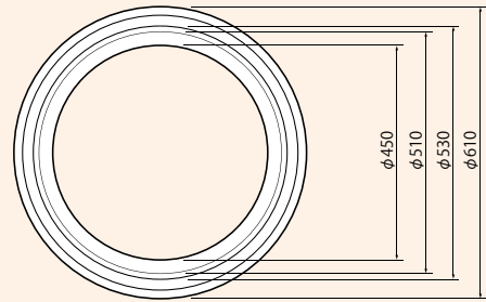
上部側塊 (T-6)
