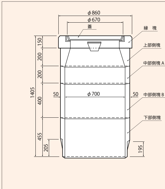
組立図 汚水
