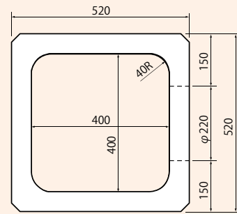
下部側塊
