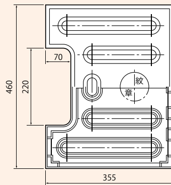
蓋(铸铁製)
