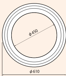
リング (T-14)
