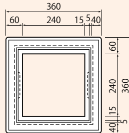
雨水枡1号
