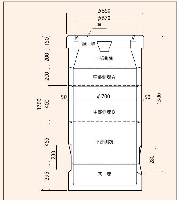
組立図 雨水
