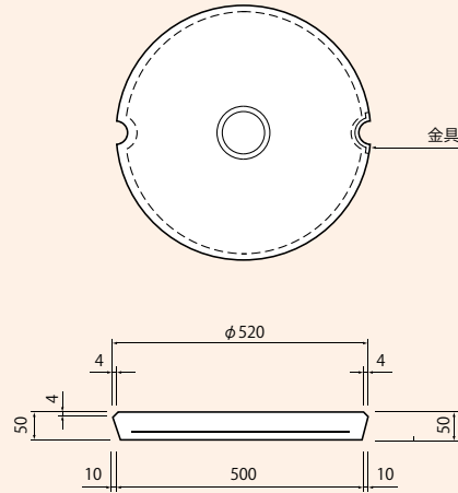
上部側塊 (T-6)
