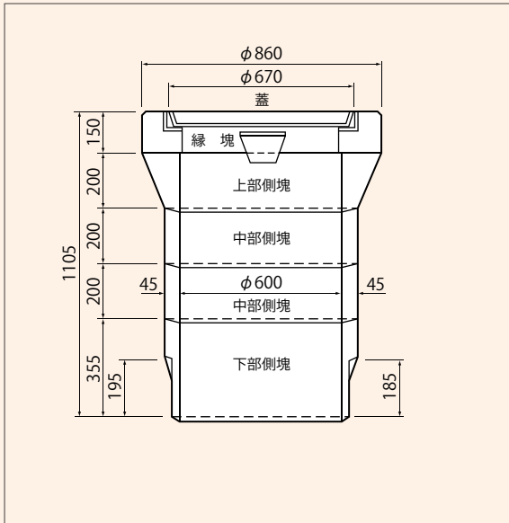
組立図 汚水
