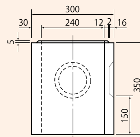
雨水枡1号
