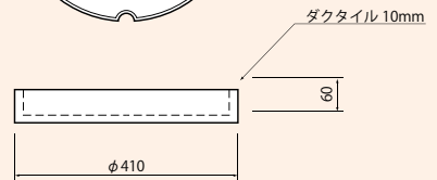
蓋 (T-6)
