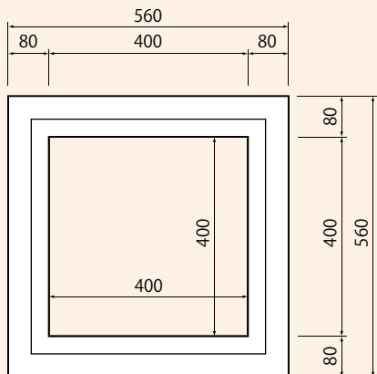
上部側塊
