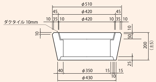
上部側塊 (T-14)
