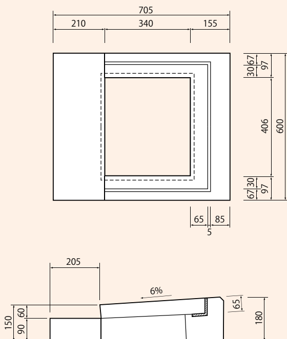
街渠柵縁塊 頭なし (155・205A)
