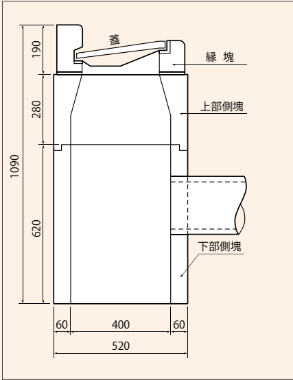
組立図
