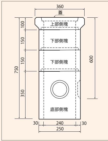
組立図
