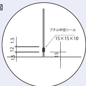
継手金物詳細図
