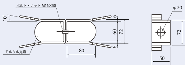
継手金物詳細図
