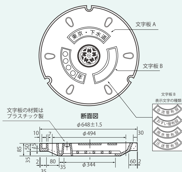
人孔コンクリート蓋(φ600用都型)
