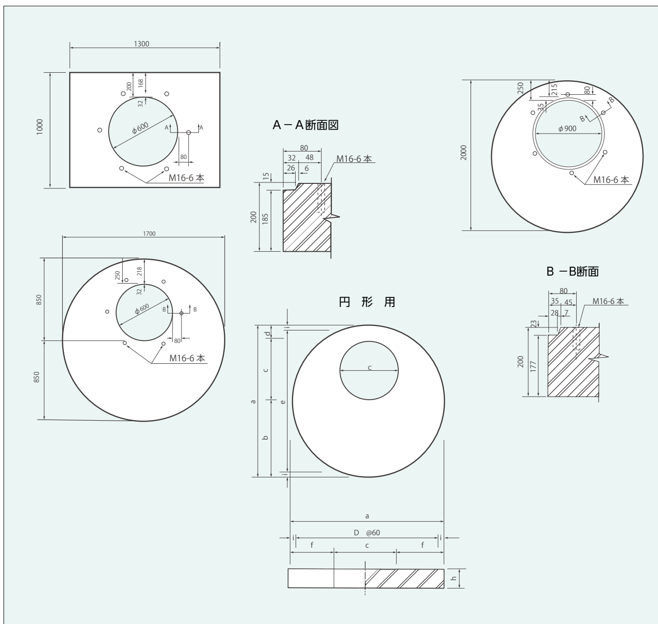
人孔床版塊(円形)
