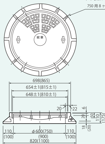
铸铁製人孔口環及びふた
