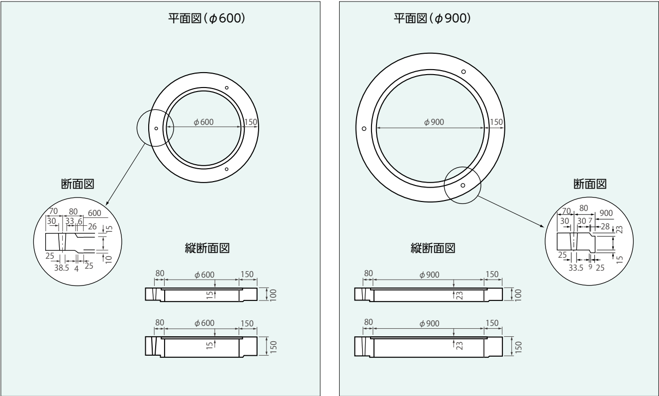
都型調整ブロック 600用・900用
