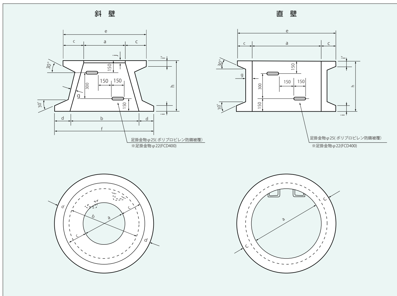
下水道用マンホール側塊
