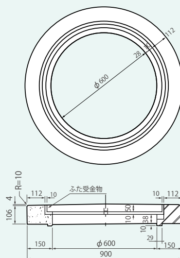
人孔口環(φ600用都型)
