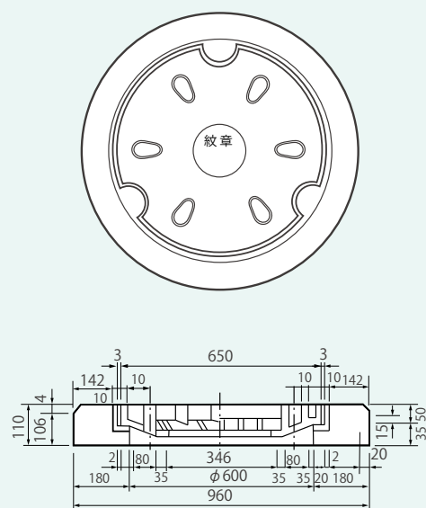
装鉄製人孔口環及びふた
